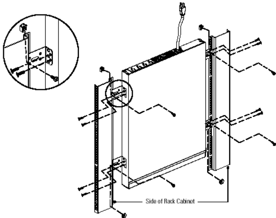
Рисунок 9. Установка Zero-U
